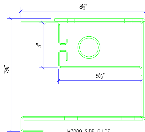
M3000 SIDE GUIDE
