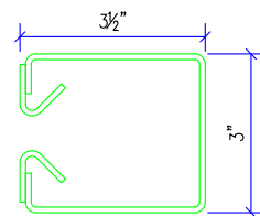
M2500 SIDE GUIDE
