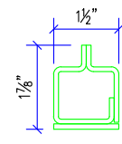
M2500 BOTTOM BAR
