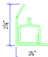
M2500 EGRESS BOTTOM BAR
